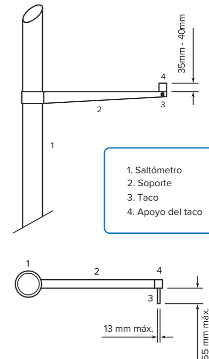
Soporte de apoyo al listón (Reglamento IAAF)
